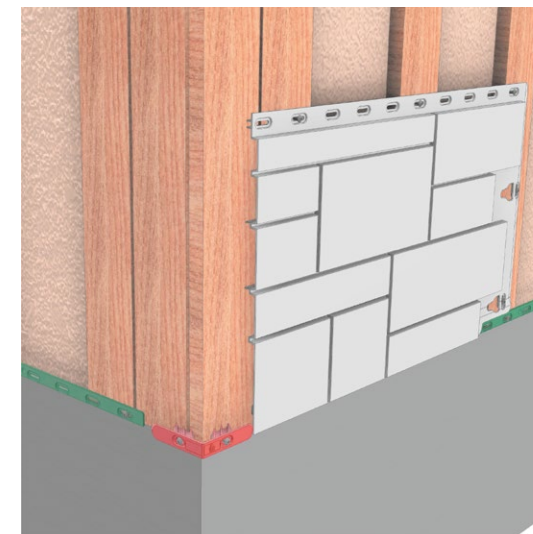
Рис. 18 Монтаж первой панели
