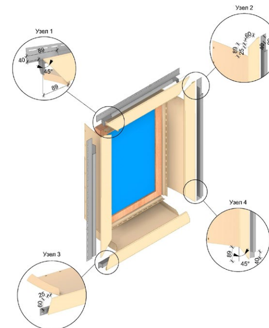
Рис. 13 Обрамление оконного проёма при универсальном околооконного профиля с соответствующим J-профилем (таблица 4).
