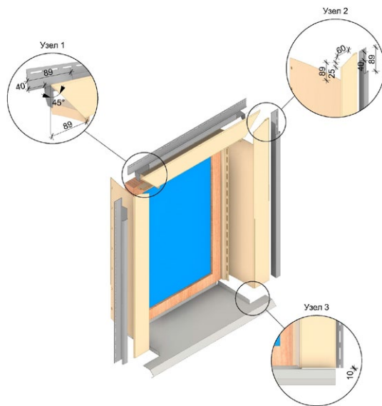
Рис. 14 Обрамление оконного проёма при универсального околооконного профиля с соответствующим J-профилем (таблица 4) при наличии металлического отлива.
